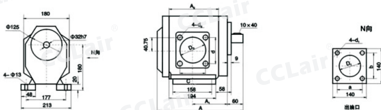
CB-B700斜齿大排量型号规格
