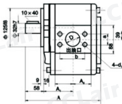
CB-B160~400斜齿大排量型号规格
