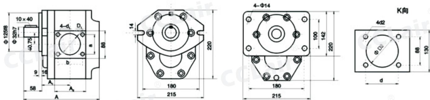
CB-B450~550斜齿大排量型号规格
